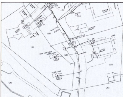
Bild 7 Werkplan
