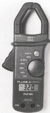
Universelle Echtheftiv-(True-RMS)-Strommesszange
