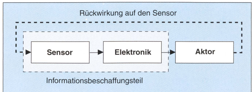
Bild 10 Geregeltes Mikrosystem
