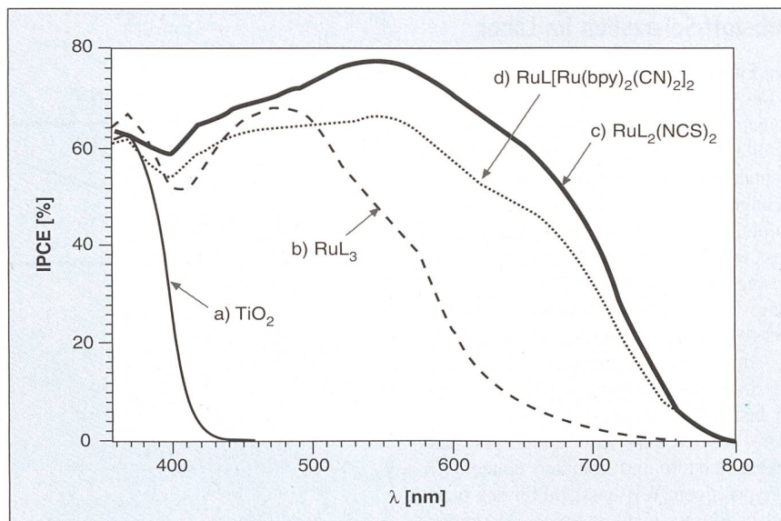
Bild 4 Aktionspektren nanokristalliner Farbstoffzellen
