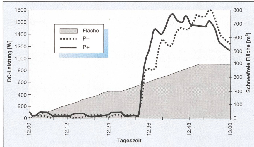
Bild 7 Verlauf der DC-Leistung während der Schneerräumung
