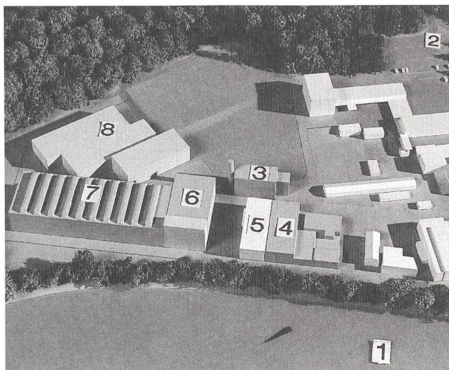
Zentrales Zwischenlager Würenlingen (Modellaufnahme).
