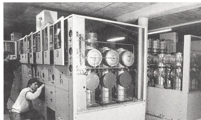
Das Besondere der grössten Mittelspannungs-Schaltanlage der Welt ist die einpolige Kapselung der Sammelschienen und Vakuumröhren.
