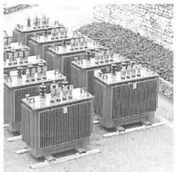
Dreiphasen-Verteiltrans- formatoren 1000 kVA; Typ A1000 16,5 ± 0,5/0,412 kV
