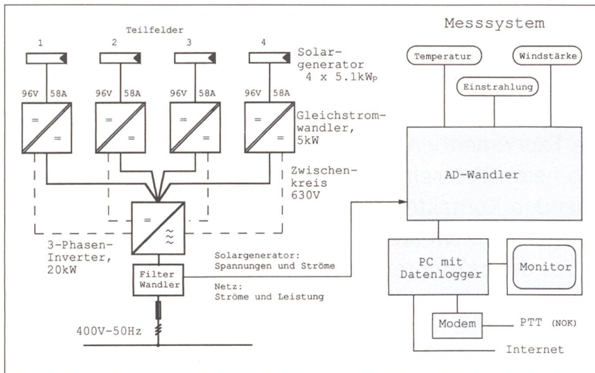
Bild 2 Prinzipschaltbild der Anlage.
