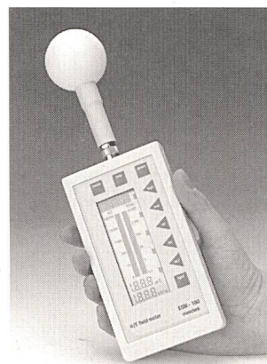
Feldstärkemessgerät ESM-100
