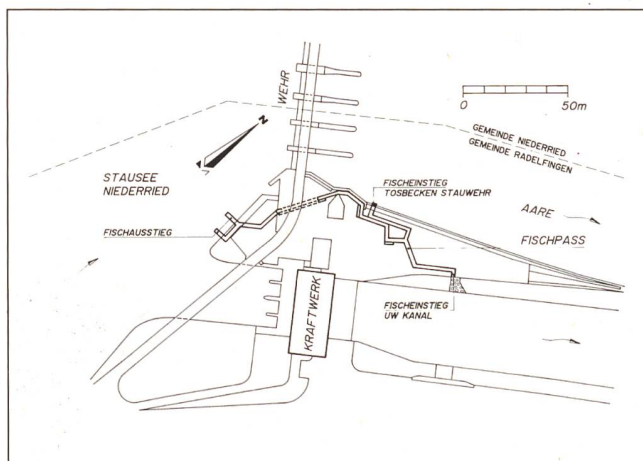
Bild 5 Kraftwerk Niederried-Radelfingen mit Fischpass (Lageplan).
