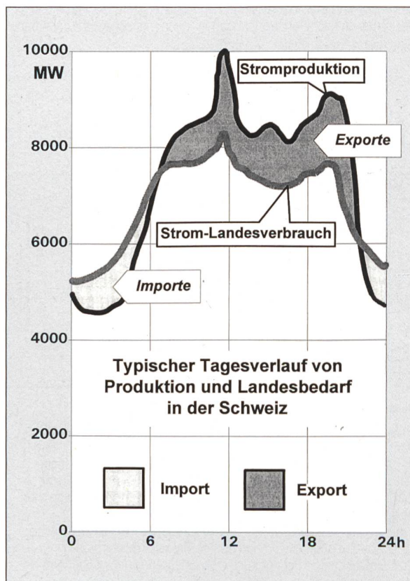
Bild 20 Lastgangkurven.
