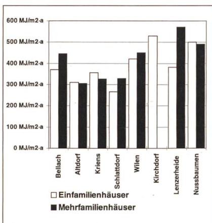
Bild 45 Schwankungen der Energiekennzahlen.
