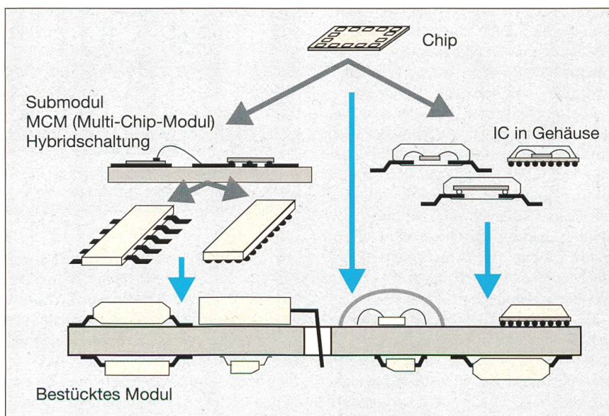
Bild 2 Aufbau- und Verbindungstechnik
