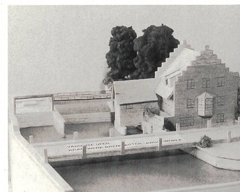
Modellaufnahme des Kleinwasserkraftwerks Bremgarten-Bruggmühle: Das 5 Mio. Franken teure Kraftwerk kann nun gebaut werden. Das AEW will die Anlage im August 1998 in Betrieb nehmen.
