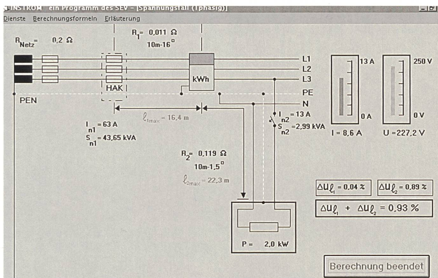
Bild 6 Simulation Spannungsfall
