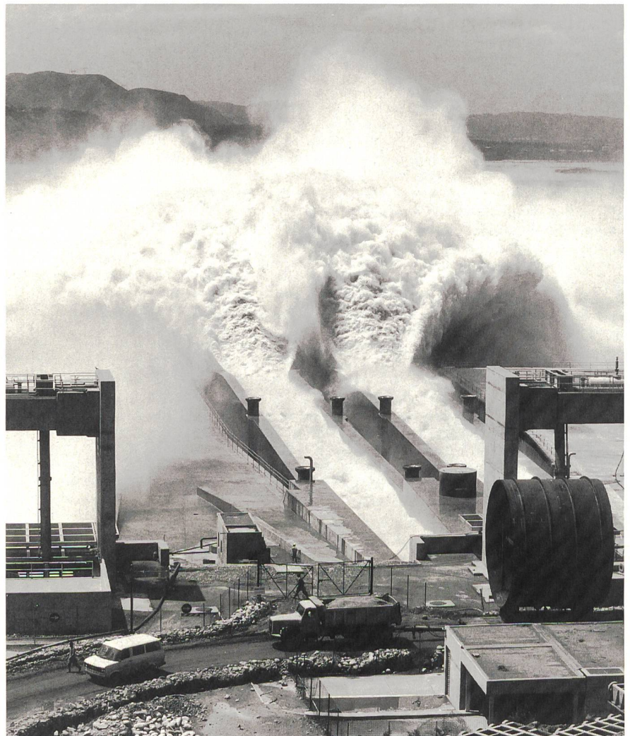
Asien hat mit 3 600 000 GWh/Jahr das grösste Wasserkraftpotential: Kraftwerk Tarbela (Pakistan; Photo Sulzer Hydro).
