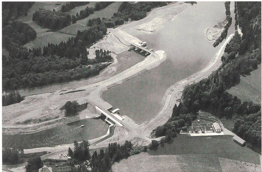
Wasserkraft unterliegt in Europa starken Beschränkungen (Lechstaustufe 8 bei Kinsau/Bayern; Photo BAWAG).
