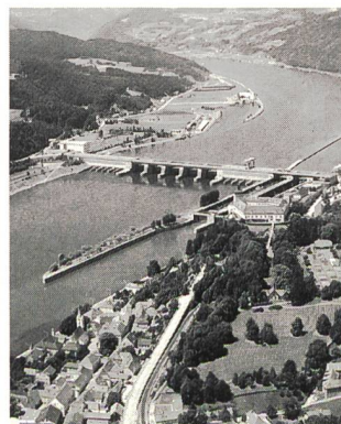
Donaukraftwerk Ybbs-Persenbeug – Symbol des österreichischen Wiederaufbauwillens vor 50 Jahren.
