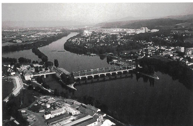
Die Rheinkraftwerke Augst (rechts, Schweiz) und Wyhlen (Deutschland) konnten aufgrund neu erteilter Konzessionen erneuert und ausgebaut werden.
