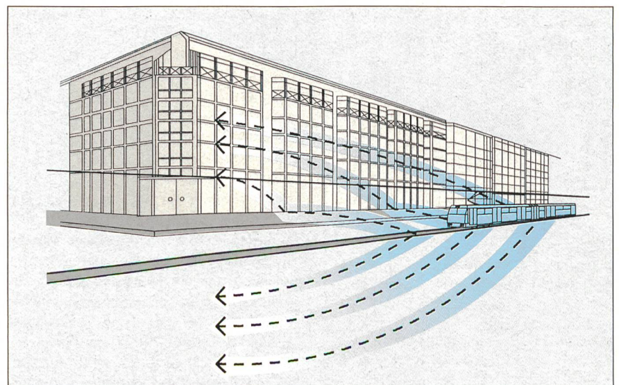
Figure 2 Courant de traction de retour pour les modes d'alimentation par ligne de contact simple selon figure 1
