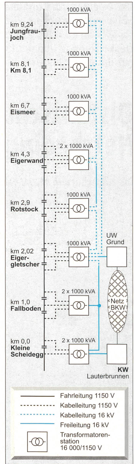
Bild 1 Energieversorgung des Fahrleitungsznetzes der Jungfrauochbahn
