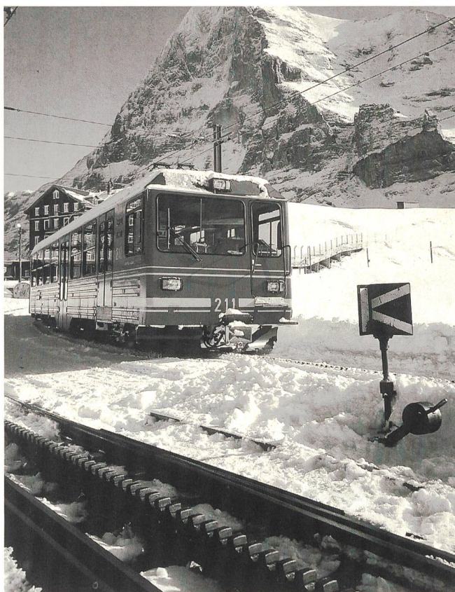
Bild 2 Doppeltriebwagen des Typs BDhe 4/8 der Jungfrauabahn
