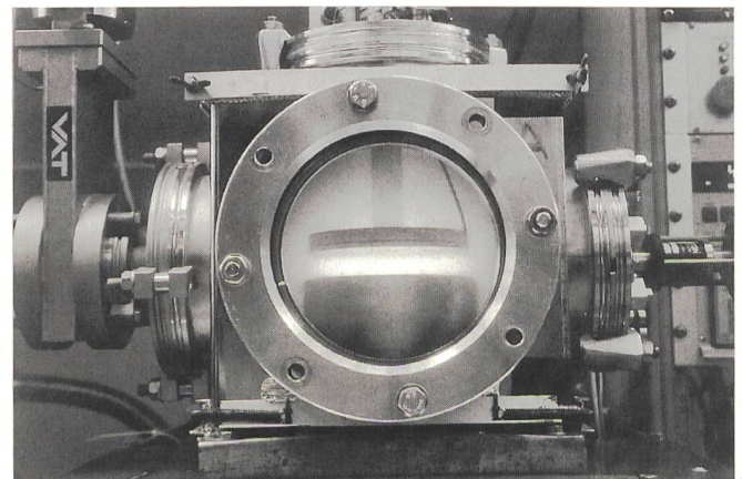
Bild 6 Blick in einen Labor-Parallelplattenreaktor
