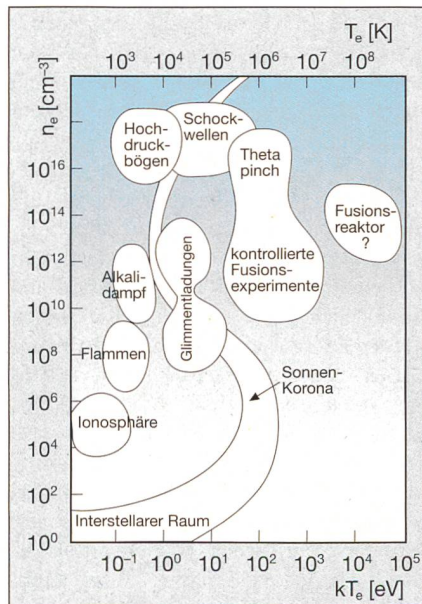
Bild 1 Überblick über Plasmen in Funktion der Elektronenenergie (Temperatur) und der Anzahldichte der Elektronen pro Kubikzentimeter im Plasmavolumen
