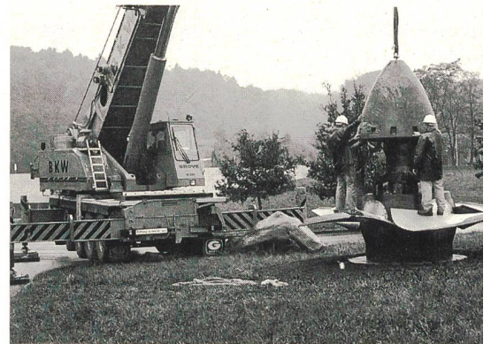
Mit neu entwickelten Rohrturbinen wird Leistung des Wasserkraftwerkes Bannwil um 7,6% gesteigert. Das Bild zeigt ein ausgedientes Kaplan-Turbinenrad. Foto: BKW
