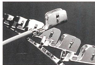
Aufsteck-Erdungsclips von Molex
