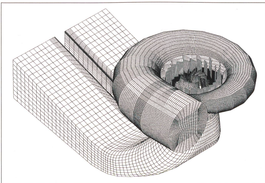
Bild 1 Erstmals konnte eine komplette Francisturbine rechnerisch simuliert werden. Hier das Rechenetz mit Spirale, Stützschaukelring, Leitschaukeln, Laufrad und Saugrohr (500 000 Knoten).
