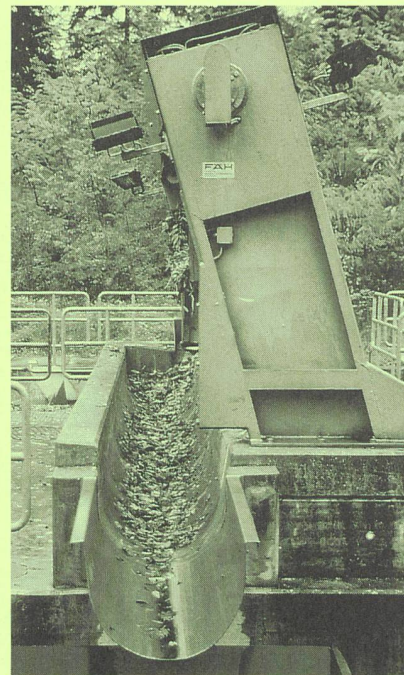
Aus der Verbandschrift 58: Entsorgung von Geschwemmel. Technik – Kosten – Zukunft. Stationäre Seilmaschine, Spülrinne.
