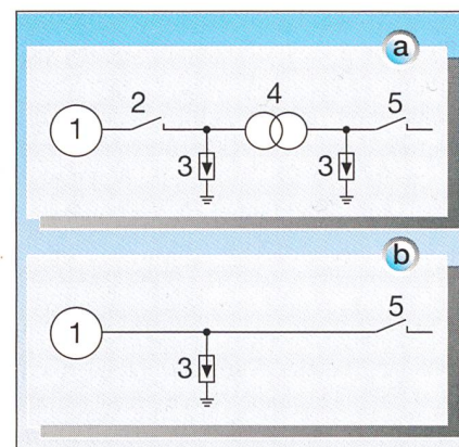
Bild 1 Schema eines konventionellen Kraftwerks mit Aufwärtstransformator (a) und gleiche Anlage bei Verwendung der neuen Technik (b)
