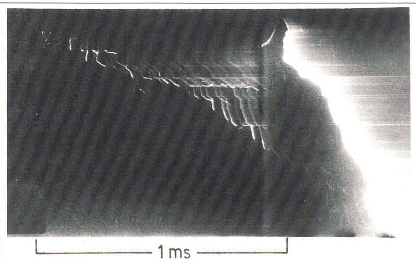
Bild 4 Schmierbildaufnahme eines negativen Abwärtsblitzes an der Turmspitze San Carlo
