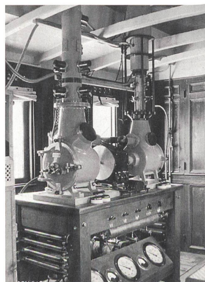
Bild 2 Oszillographen in Bergrers Messwagen
