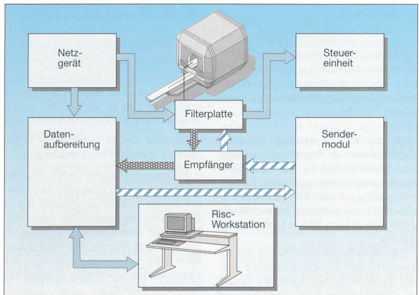
Bild 5 Blöckschaltbild eines MRS (Bruker Medspec Avance MR System)
