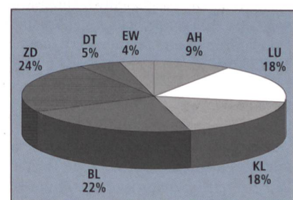
Bild 6 Aufteilung des Elektrizitätsverbrauchs nach Verwendungszweck, gewichtet nach absolutem Verbrauch (AH: Arbeitshilfen, LU: Lüftung, KL: Kälte, BL: Beleuchtung, ZD: Zentrale Dienste, DT: Diverse Technik, EW: Elektrowärme).
