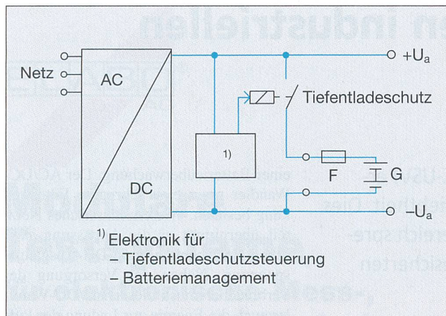
Bild 2 Blockscha eines Online-DC-USV-Systems (Quelle: J. Schneider Elektrotechnik)
