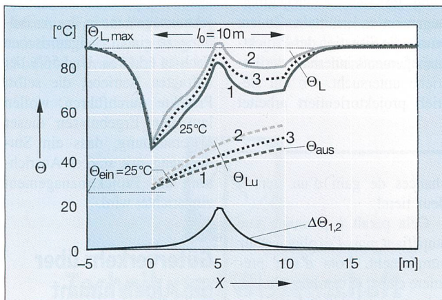
Bild 4 Temperaturverteilungen im Kreuzungsbereich für eine Anordnung nach Bild 1 für unterschiedliche Rohrendurchmesser d_i . 1: Rohrendurchmesser 100 mm; 2, 3: Rohrendurchmesser 70 mm; 1, 2: Auslasshöhe h_z = 0 m; 3: Auslasshöhe h_z = 2,5 m; Kühlabschnittslänge l_0 = 10 m; Luft-Eintrittstemperatur \Theta_{\text{ein}} = 25^\circ\text{C} ; sonstige Parameter wie in Bild 2
