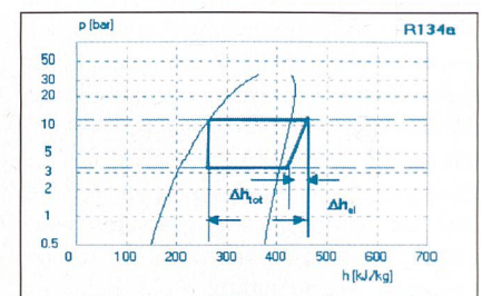
Bild 3 Kreisprozess ohne Unterkühlung; Leistungszahl Verdichter: \Delta h_{tot} : \Delta h_{el} = 4,7 .
