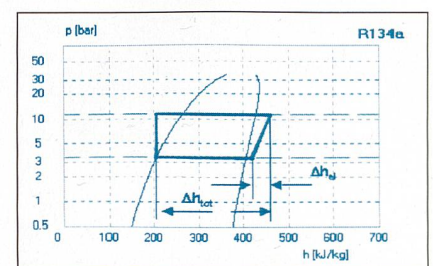
Bild 4 Kreisprozess mit 40 K Unterkühlung; Leistungszahl Verdichter: \Delta h_{tot} : \Delta h_{el} = 6,2 .
