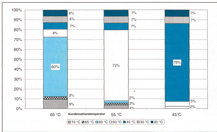
Bild 2 Aufteilung der Leistungsanteile bei verschiedenen Vorlauftemperaturen.
