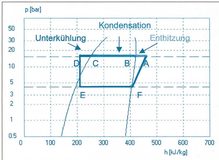
Bild 1 Darstellung von Entwärmung, Kondensation und Unterkuhlung im Kreisprozess.
