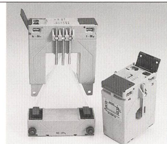
Kabelumbauwandler
