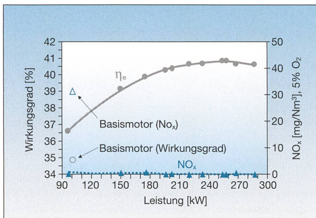
Bild 5 Wirkungsgrad in % (als Punkte) und NO x -Emissionen in mg/Nm 3 bei 5% O 2 (als Dreiecke) des Swissmotors in Abhängigkeit der Leistung in kW
