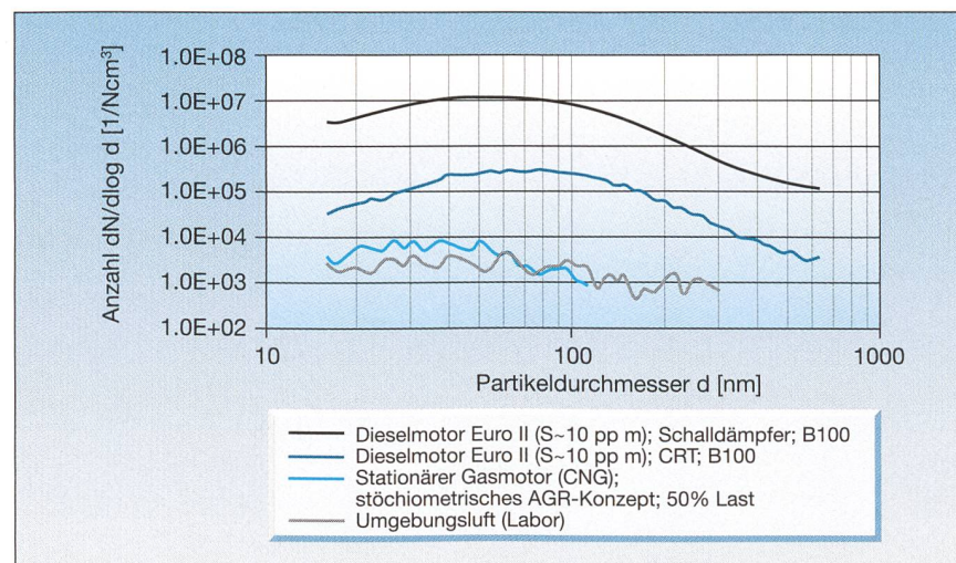
Bild 6 Partikelaustritt (jeweils Grösse und Anzahl der Partikel)
