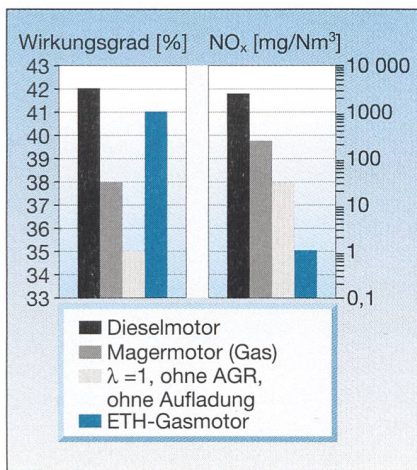
Bild 4 Wirkungsgrad und NO x -Emissionen von vier Motorkonzepten
