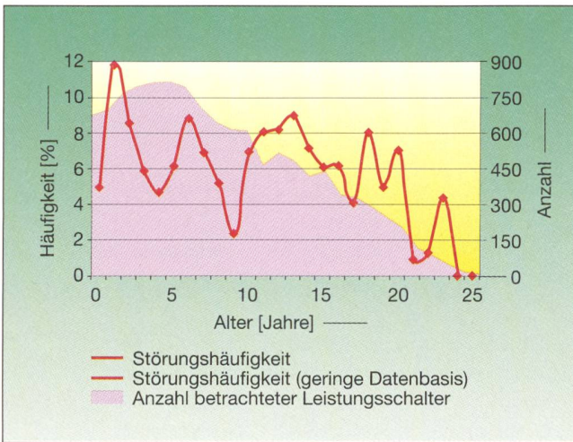
Bild 3 Fehlerhäufigkeit von SF 6 -Leistungsschaltern
