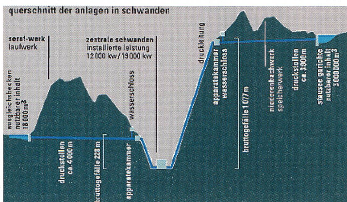
Bild 5 Wasserkraftwerke in Schwanen.
