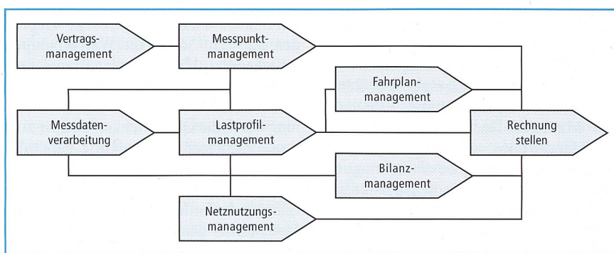
Bild 1 Für das Energiedatenmanagement relevante Prozesse des Verteilnetzbetreibers/Lieferanten.
