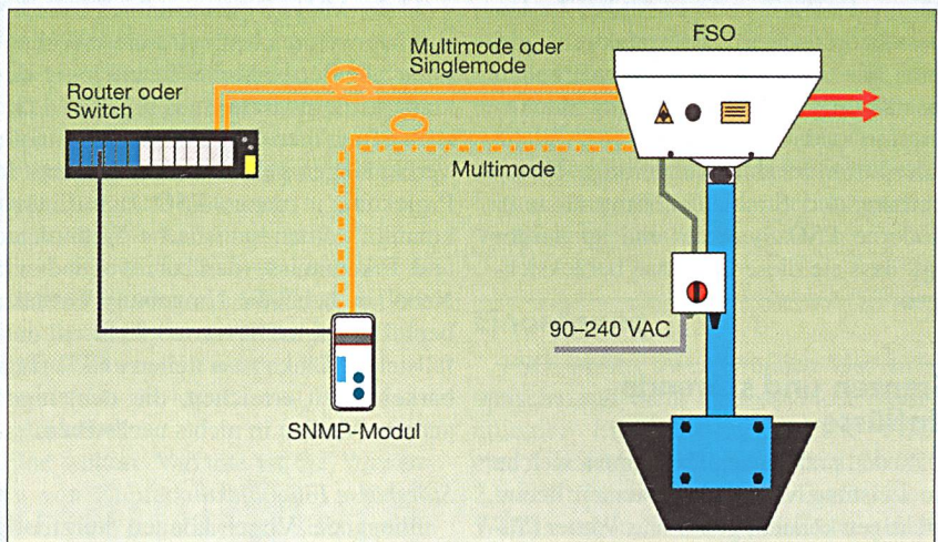
Remote Management einer FSO-Verbindung
