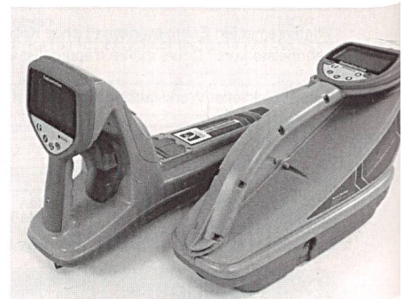
RD4000-Sender und -Empfänger von Radodetection Ein internetfähiges Ortungssystem.
