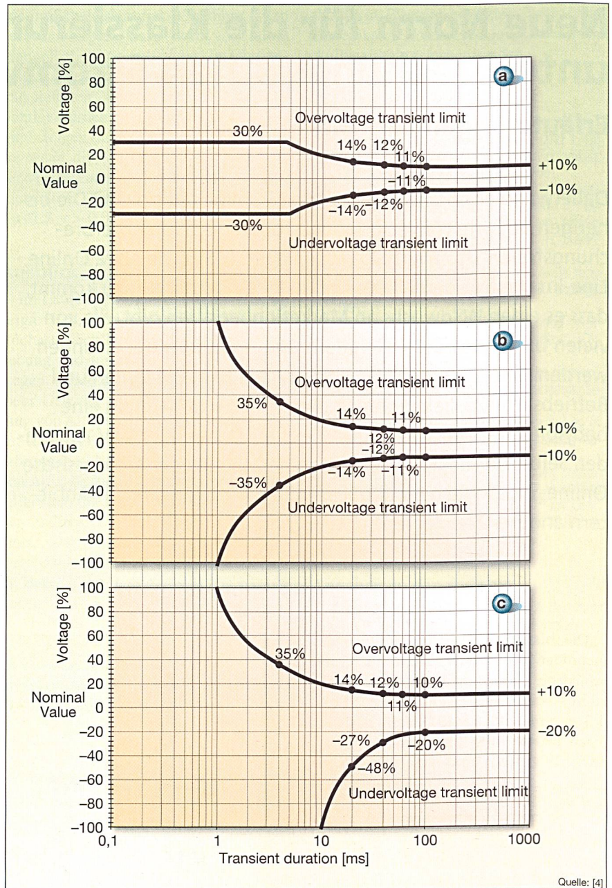
Bild 1 Dynamische Toleranzkurven des Ausgangs
