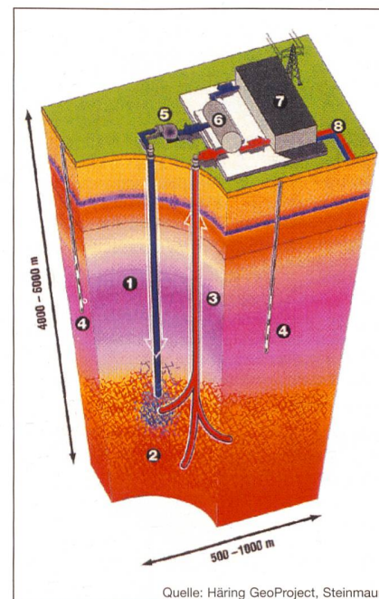
Bild 3 Schematische Darstellung des «Hot Dry Rock»-Verfahrens
