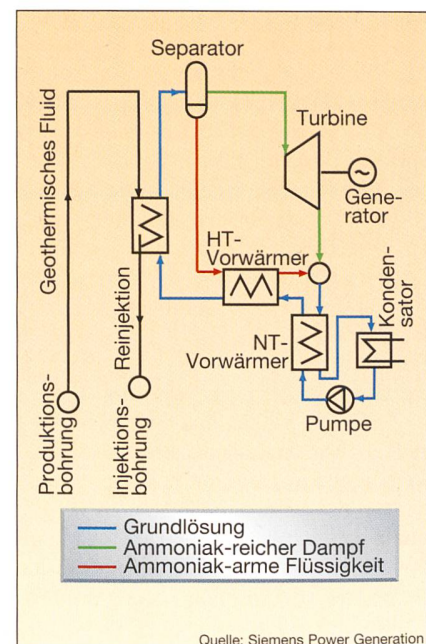
Bild 5 Blockschaftbild des Kalina-Prozesses HT: Hochtemperatur; NT: Niedertemperatur
