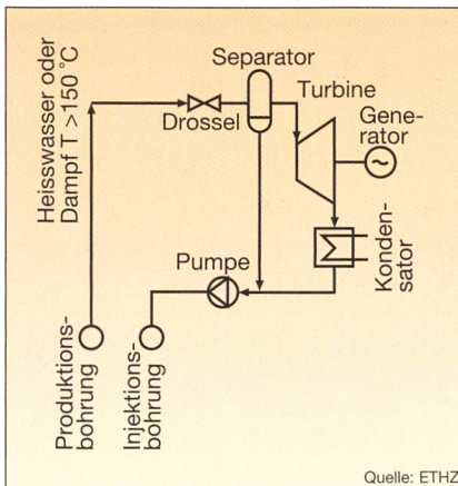
Bild 4 Blockschaftbild für die direkte Nutzung des geothermischen Fluids
