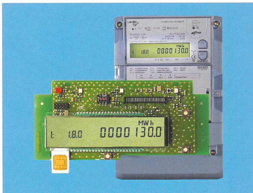
Bild 5 Cryptochip als Standardlösung.
