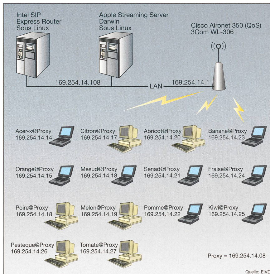
Figure 2 Plateforme de test
