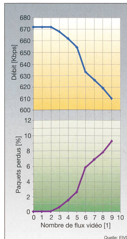
Figure 3 Performance de la vidéo sur WLAN
