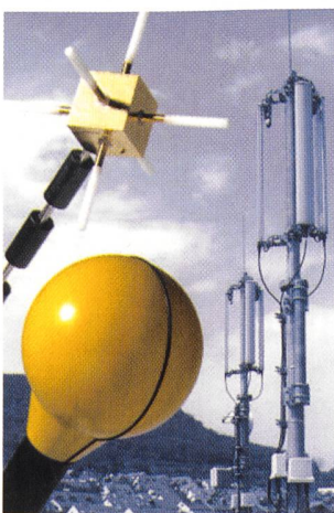
Die neue Sonde von Narda STS erfasst einen Frequenzbereich von 80 MHz bis 3 GHz
