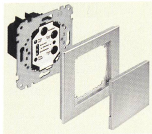
Die Brücke zwischen Instabus EIB und dem Merten-Funksystem: das Funk-Gateway UP
