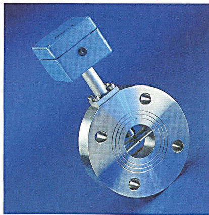
Messumformer direkt auf dem Durchflusssensor montiert; der Sensor selbst ist hier im Messrohr installiert
