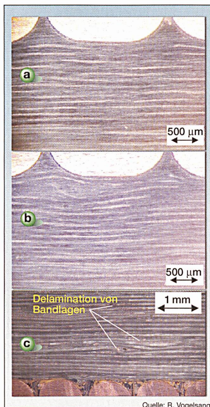
Bild 5 VPI-Wicklungsisolierung
