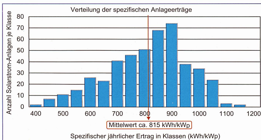
Bild 1 Der mittlere spezifische Jahresertrag der Solarstromanlagen im Jahre 2004 betrug rund 815 kWh/kW p , dank gut 5% mehr Einstrahlung immer noch leicht über dem langjährigen Mittel von 800 kWh/kW p .
