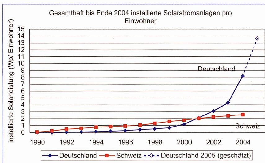
Bild 5 Mittlerweile hat Deutschland sogar Japan überholt und führt die weltweite Rangliste mit der gesamthaf installierten Solaranlagenleistung pro Kopf an.
