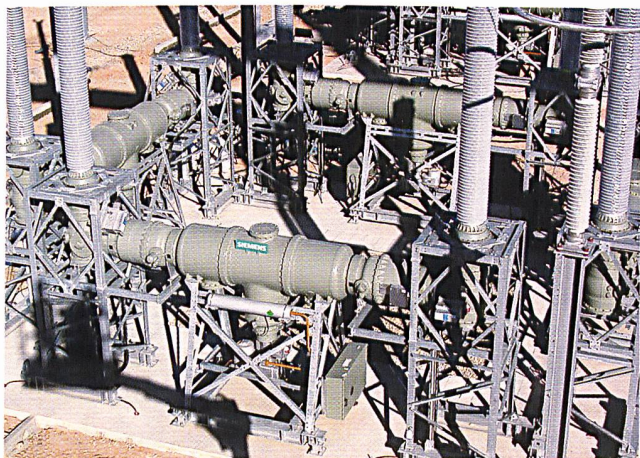
420-kV-Hochspannungs-Schaltanlage.
