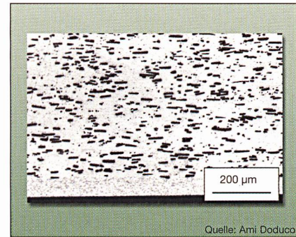
Bild 7 Längsschliff-Gefüge von Ag/C mit Anteil an Graphitfasern, an der Unterseite Schweissrücken aus Ag/Ni 10 3 )
