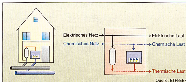
Bild 1 Symbolische Darstellung eines Haushalts, der mit Boiler und Brenner aus elektrischer (schwarz) und chemischer (blau) Energie thermische Energie (rot) erzeugt; Darstellung als Energy Hub
